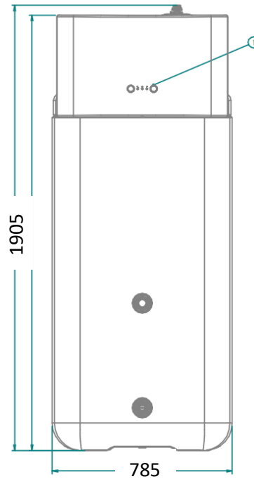
Ansicht von vorne Alle Optionen 500 l
