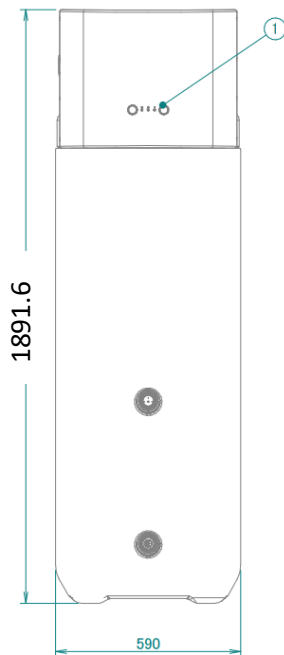
Ansicht von vorne Alle Optionen 300 l
