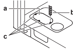
a الفتحة الكبيرة القابلة للزحف b مثقاب c نقاط للتقّب
