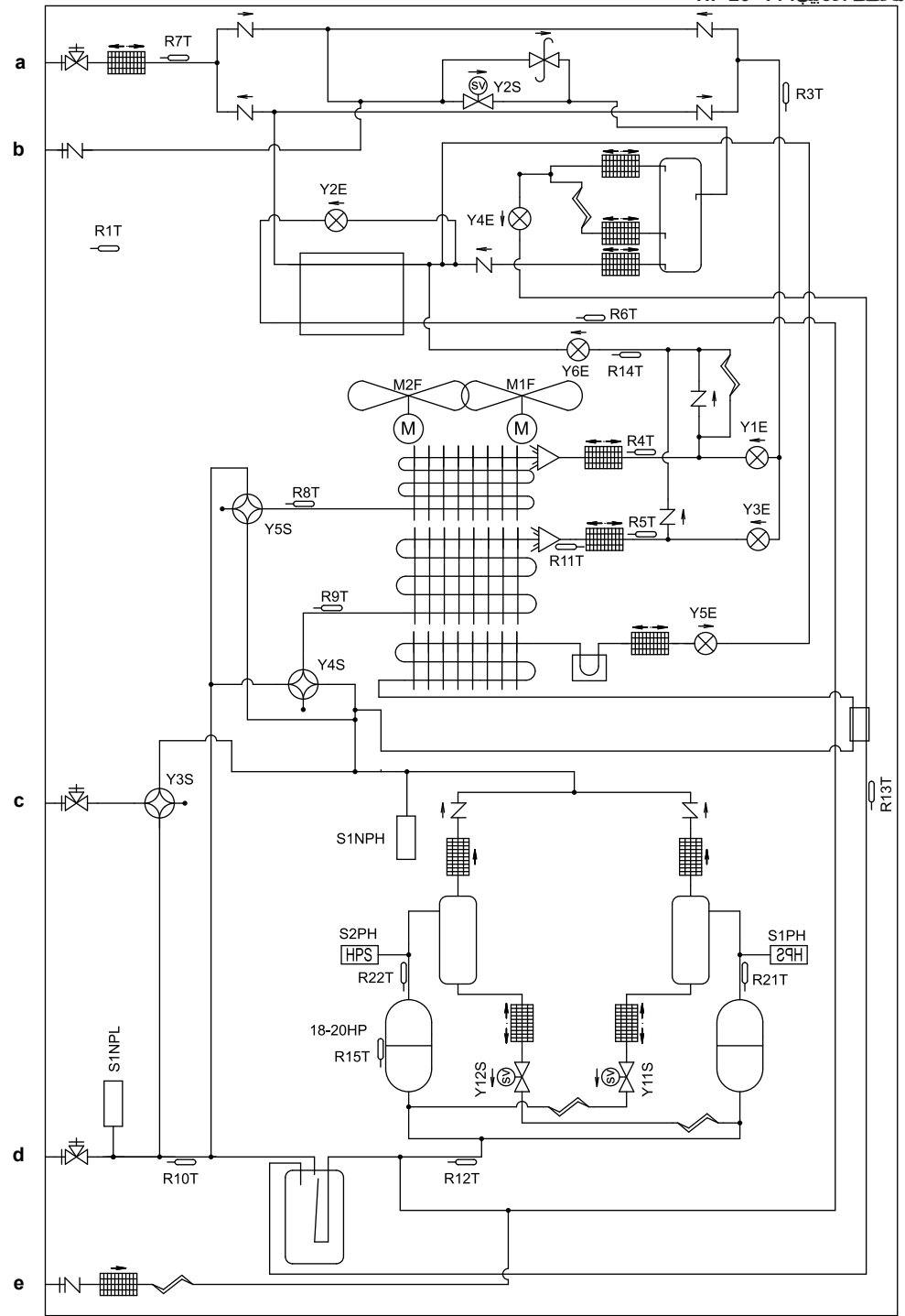
مخطط الأنابيب: HP 20~14
